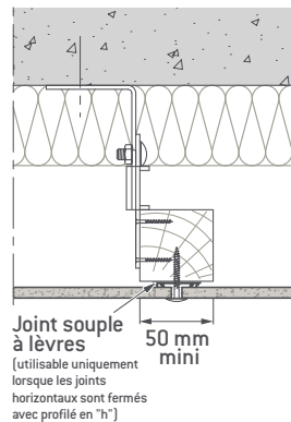
Joint horizontal fermé sur chevron intermédiaire
