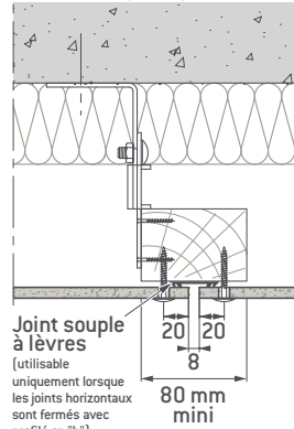
Joint horizontal fermé sur chevron principal
