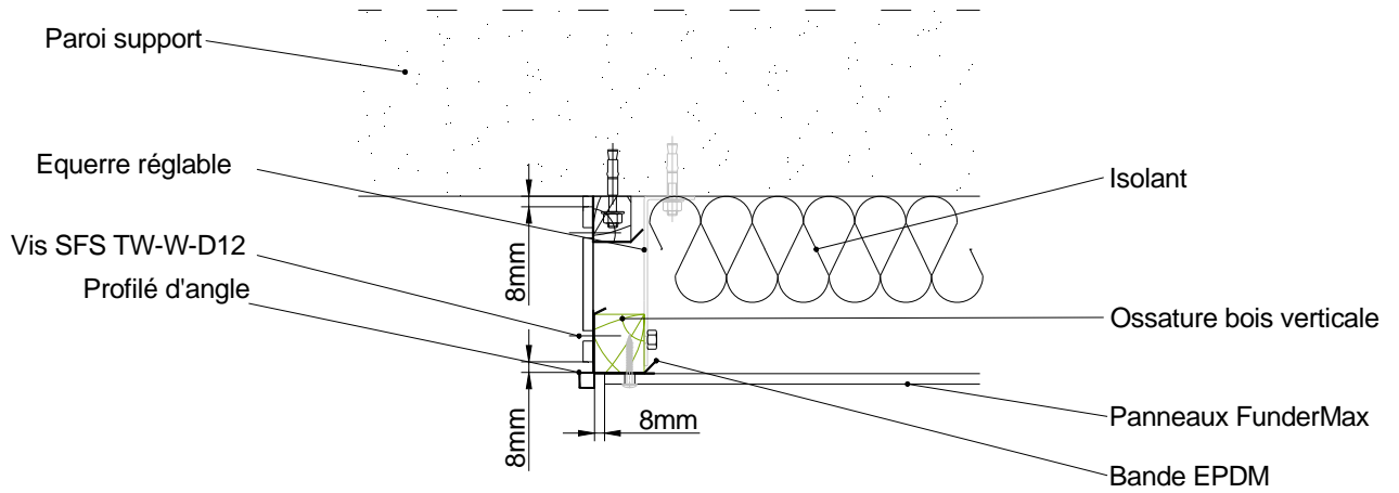
Figure 8 – Arrêt latéral en façade
