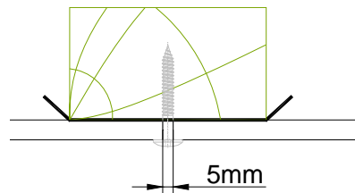
Figure 6.1 – Joint vertical à la jonction de panneaux
