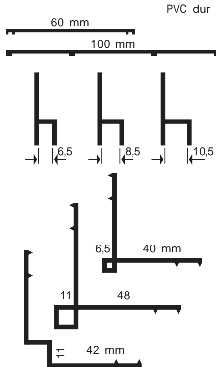
Figure 3 – Profilés complémentaires
