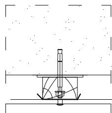
Figure 49 – Pose en zones sismiques – pose directe sur le support - Coupe horizontale
