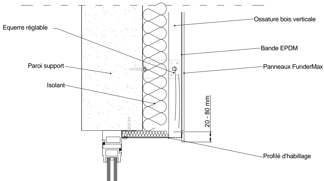
Figure 17.1 – Linteau de fenêtre
