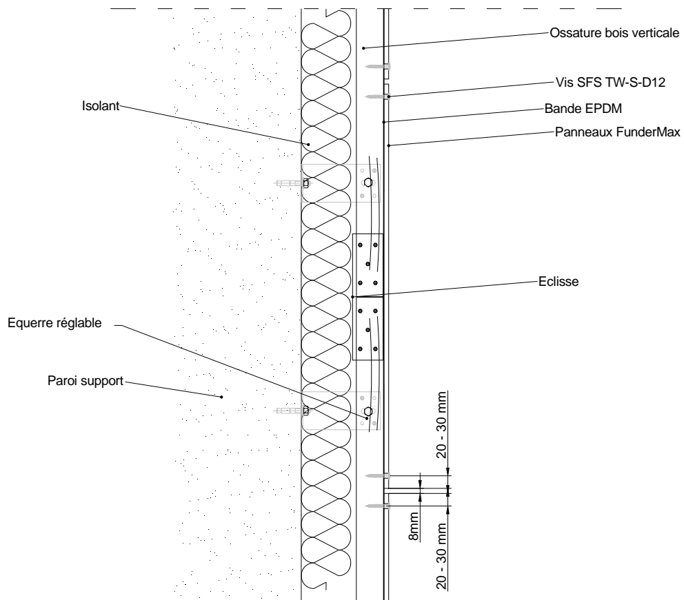
Figure 13 – Raboutage d'ossature par éclissage mécanique longueur jusqu'à 12 m
