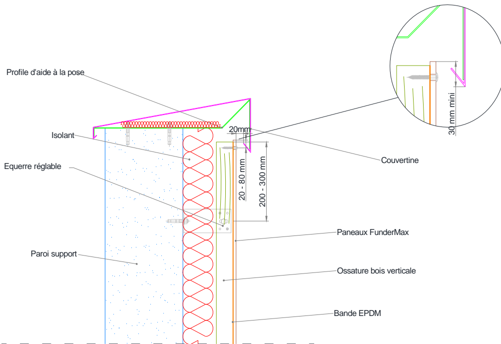
Figure 7.2 – Arrêt haut avec couvertine
