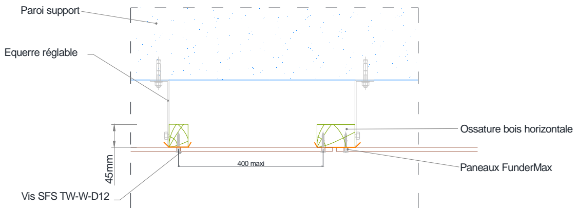
Figure 30 – Pose en sous-face – Coupe verticale sans isolant
