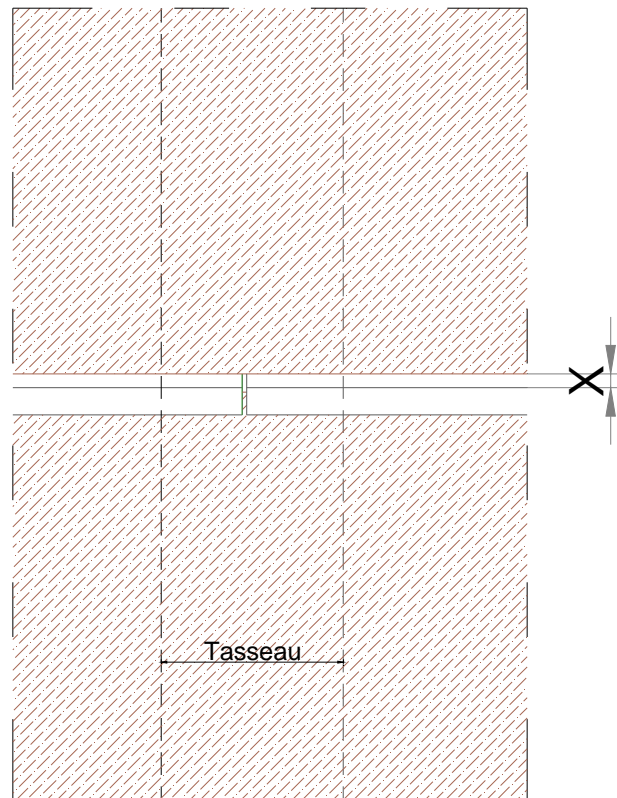
Figure 20.2 – Aboutage des profilés de fermeture des joints horizontaux sur tasseau pour COB supérieure à 10 m
