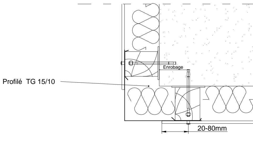
Figure 51 – Pose en zones sismiques – pose directe sur le support - Angle sortant
