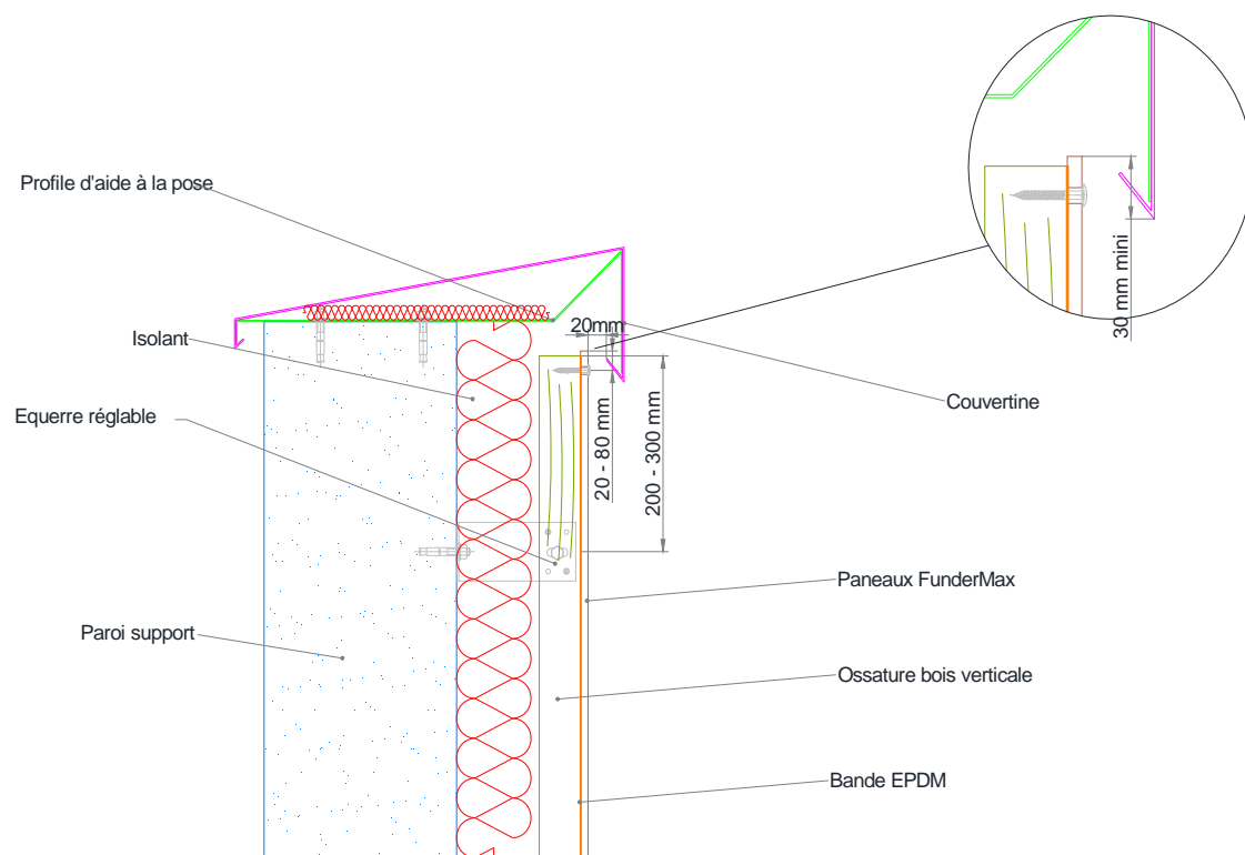
Figure 34 – Arrêt haut avec couvertine
