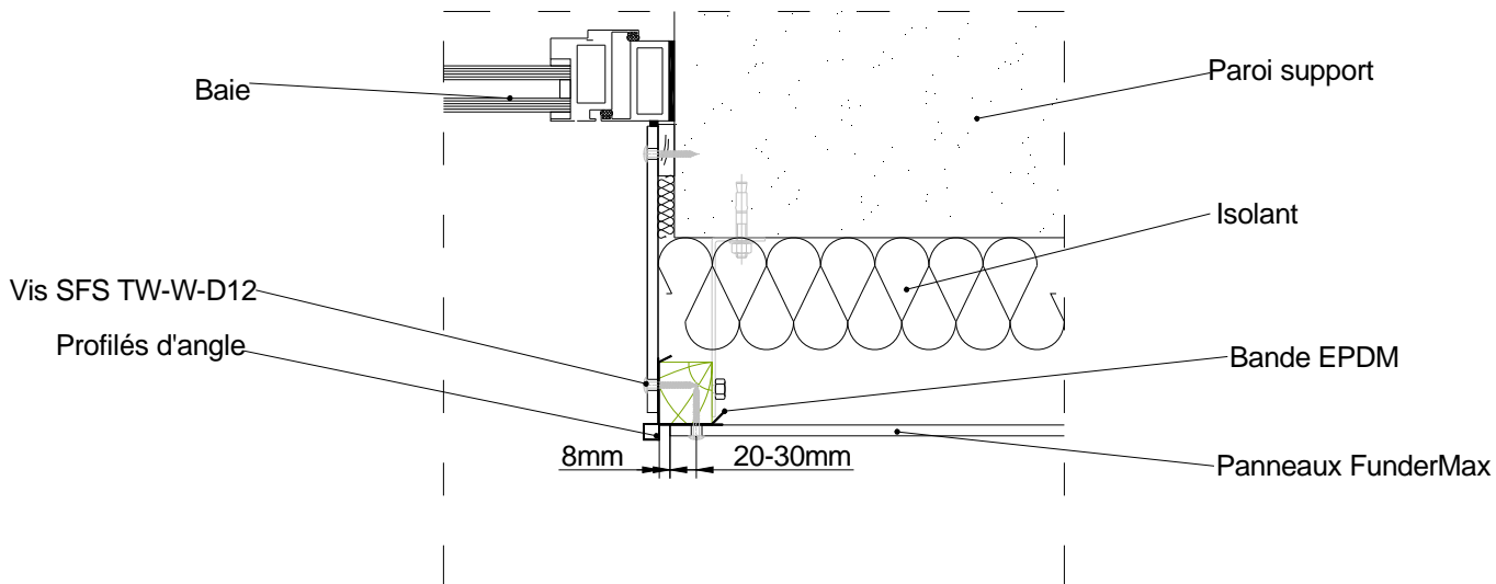
Figure 16.2 – Pose en tableau
