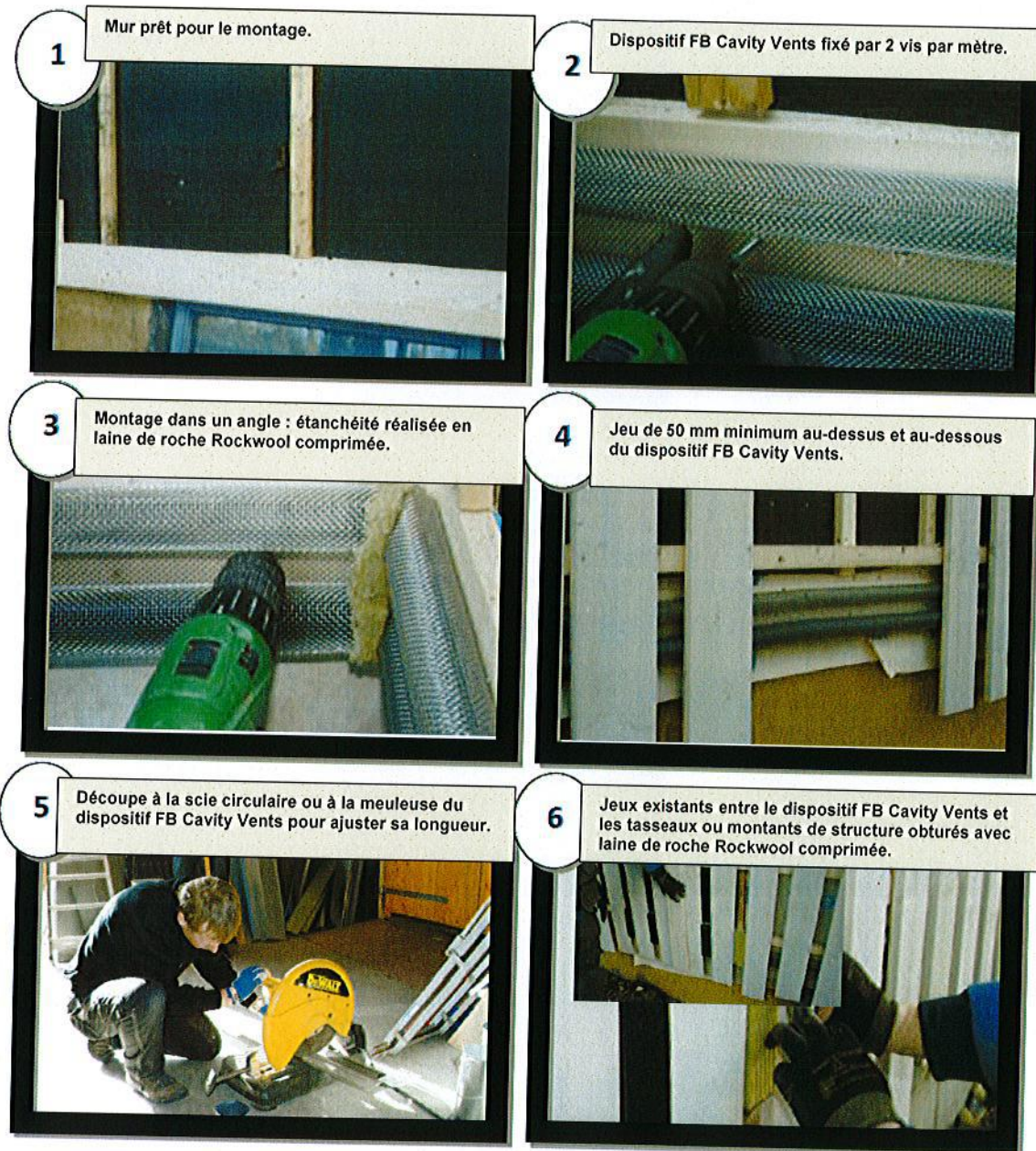
Figure 5: Détails de la mise en œuvre derrière un bardage ventilé en bois
