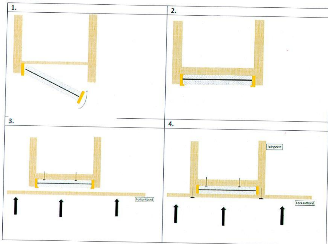
Figure 4: Montage entre deux poteaux existants
