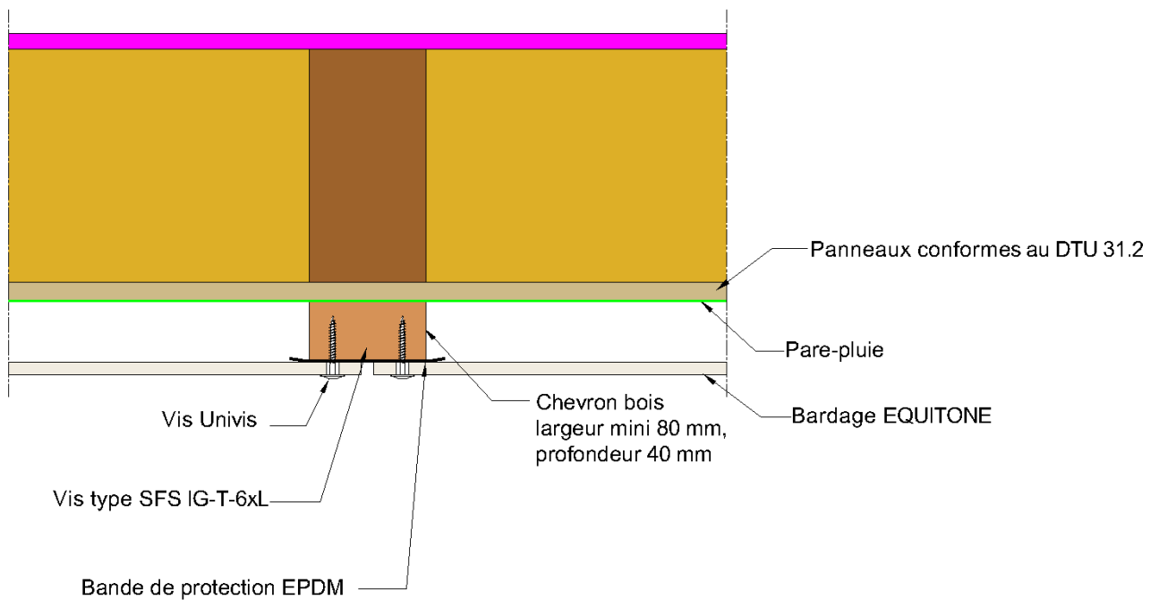
Figure 24 - Fixation sur chevron principal - Pose sur COB
