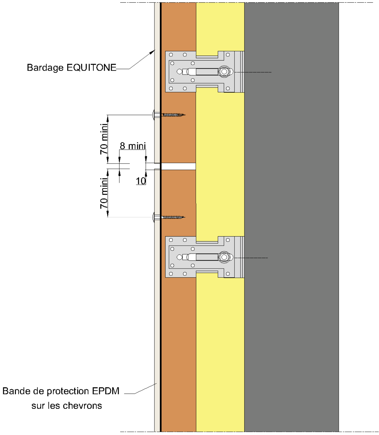
Figure 17- Fractionnement de l'ossature pour des montants d'une longueur < à 5,4 m
