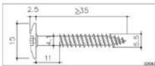
UNIVIS \varnothing 5,5 x 35 mm
