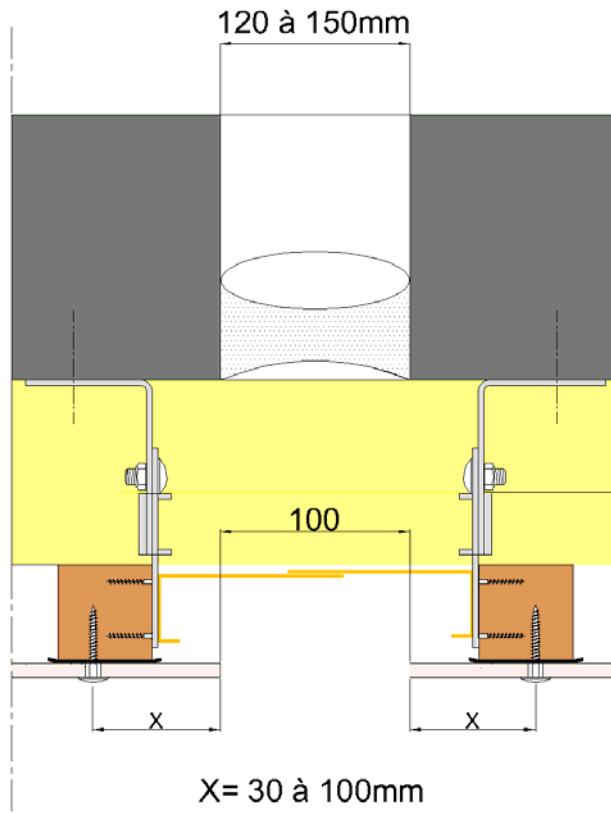
Figure 38 – Joint de dilatation de 12 à 15 cm
