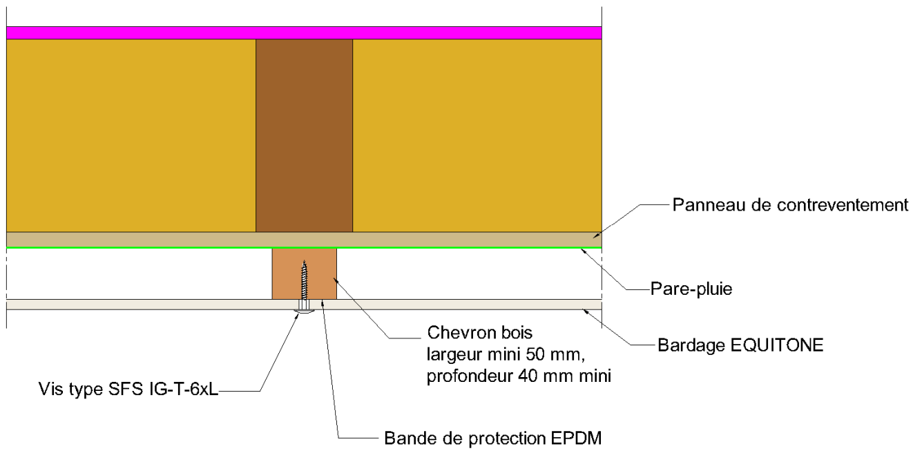
Figure 23 - Principe de fixation des chevrons – Pose sur COB
