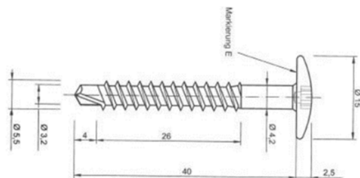
UNIVIS \varnothing 5,5 x 40 mm (DP)
