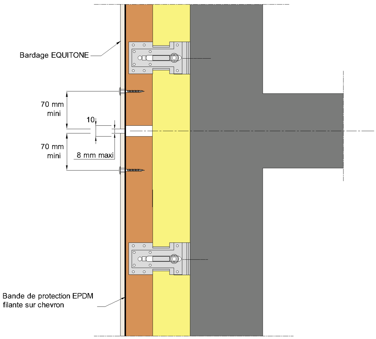
Figure 36 - Fractionnement de l'ossature bois au droit de chaque plancher
