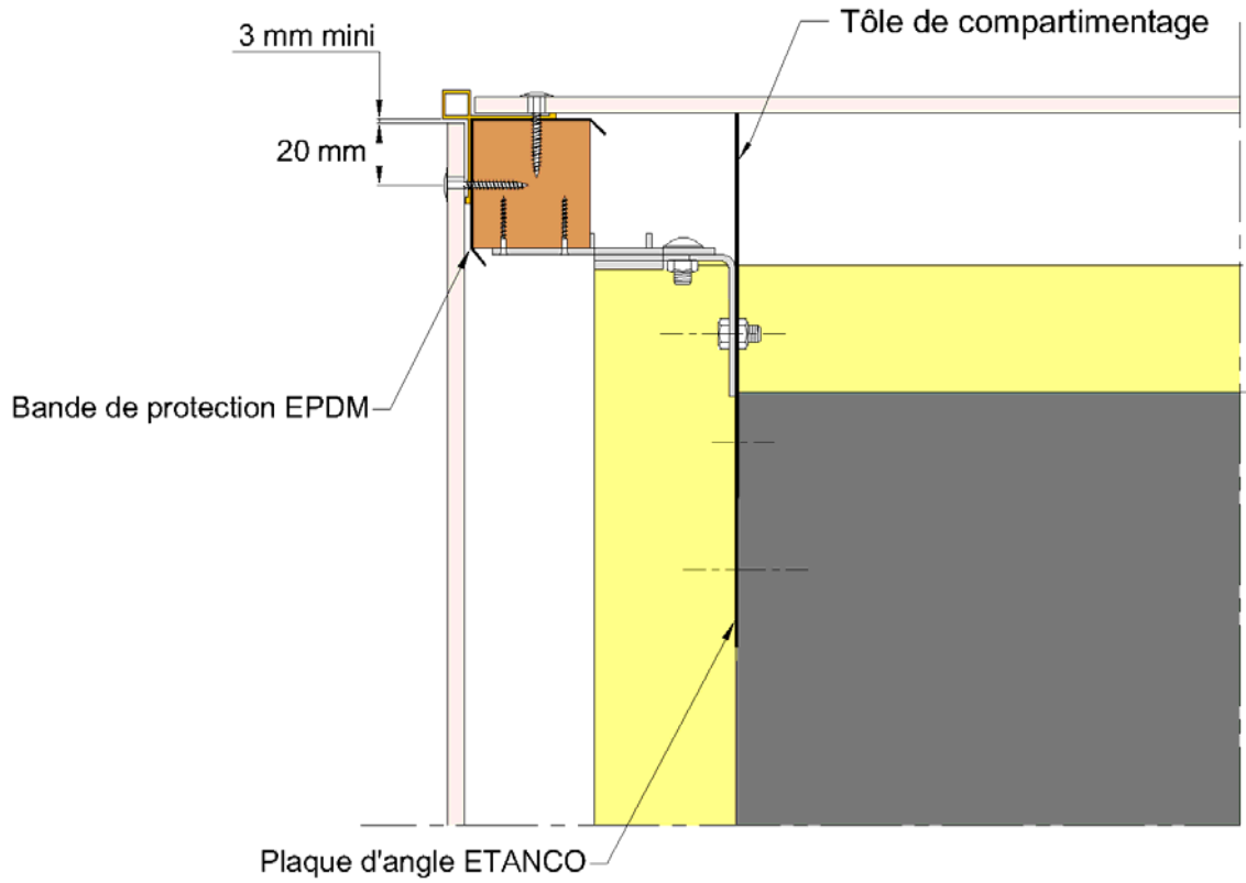
Figure 11 - Angle sortant avec profilé (bardage)
