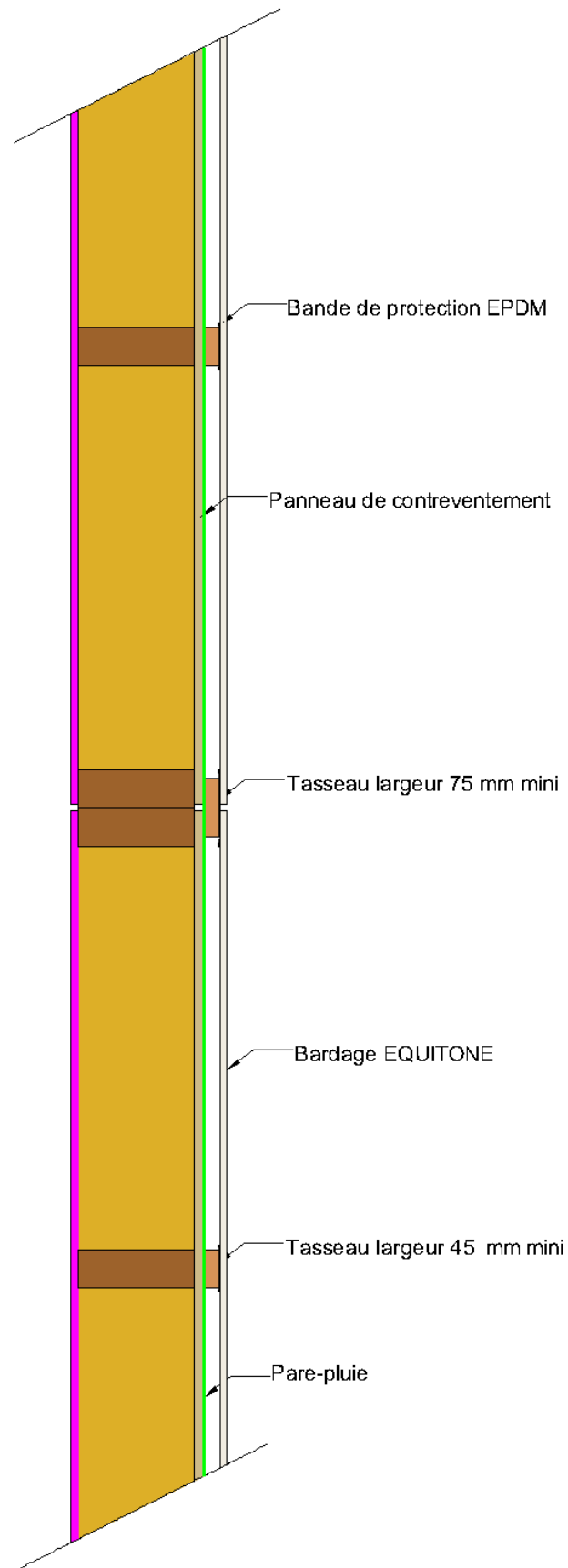
Figure 19 - Pose sur COB - Coupe horizontale
