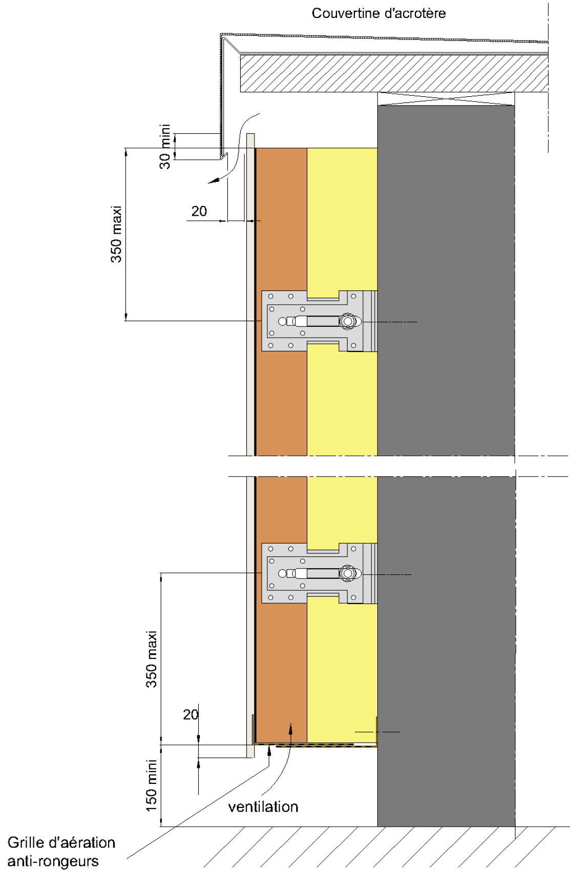
Figure 10 - Rives haute et basse
