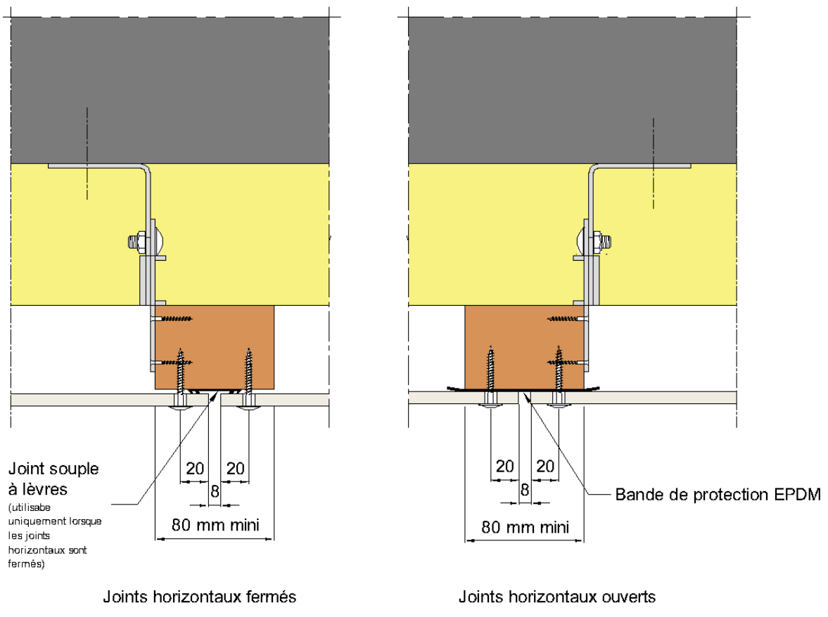
Figure 8 - Fixation sur chevron principal
