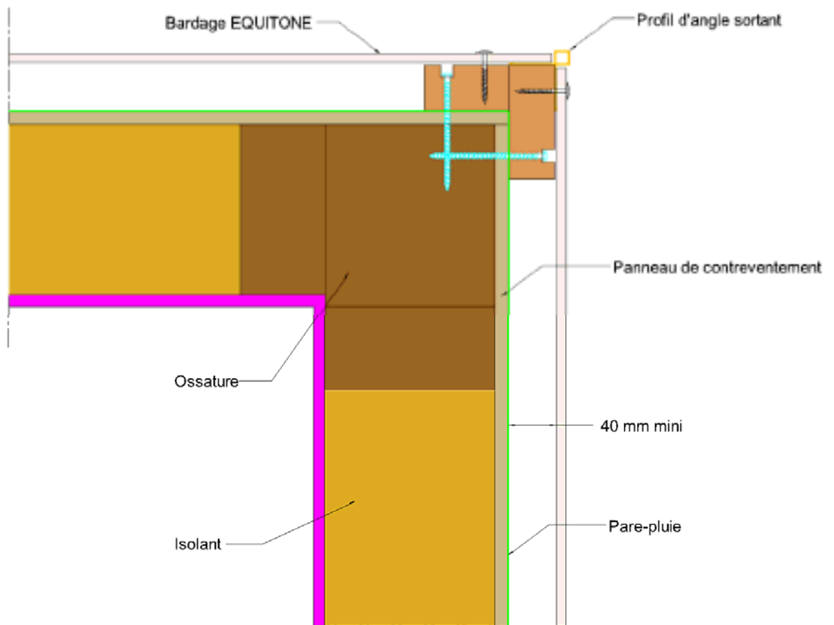
Figure 26 - Traitement de l'angle sortant - Pose sur COB
