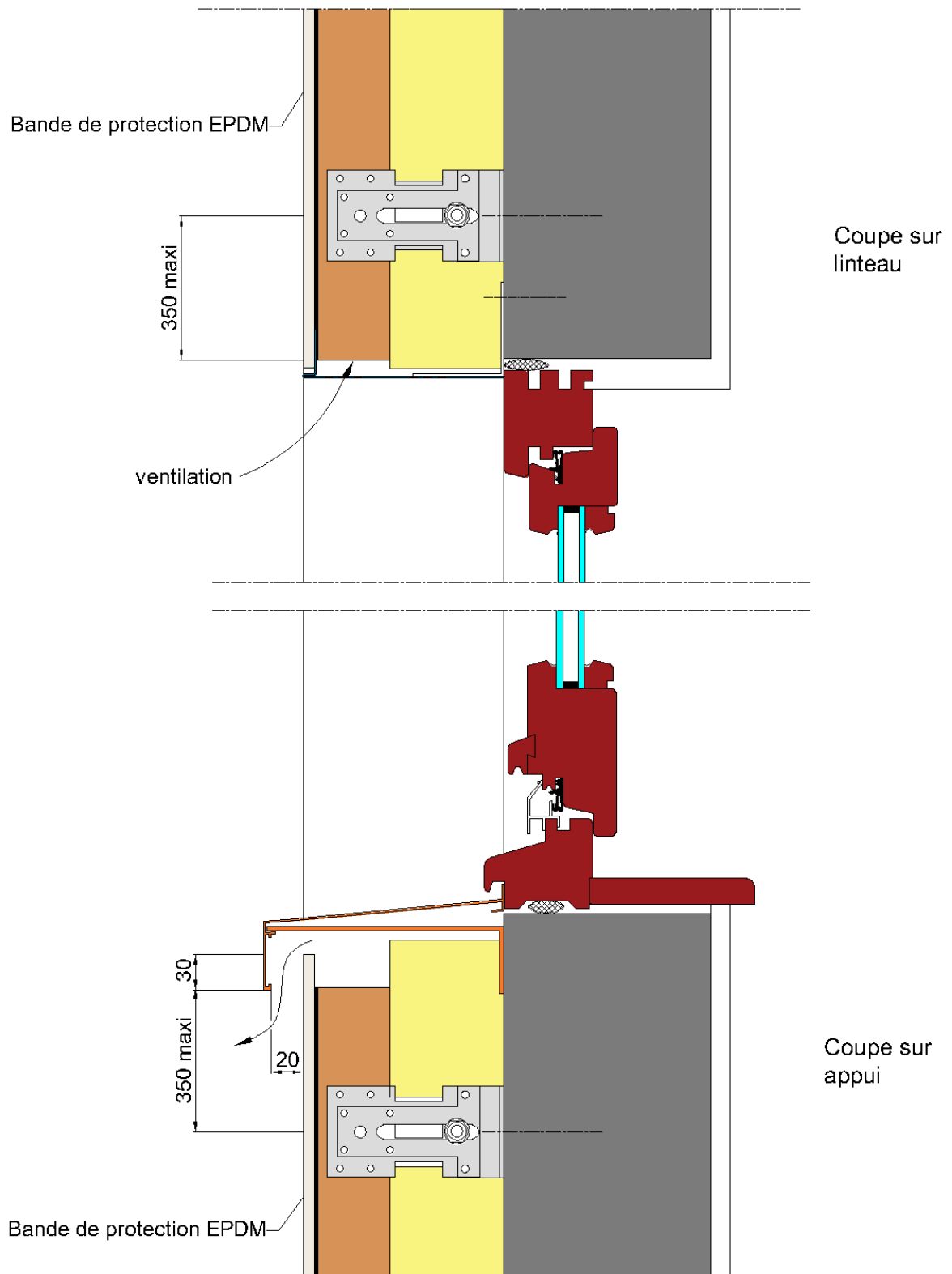
Figure 15 - Encadrement de fenêtre
