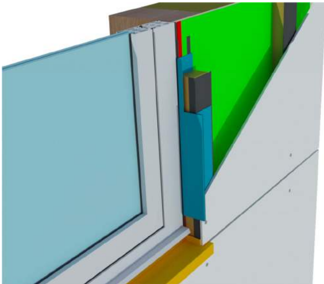
Figure 35 – Pose sur COB – Dispositions particulières du traitement des baies Menuiserie en tunnel au nu extérieur – Coupe sur linteau de baie
