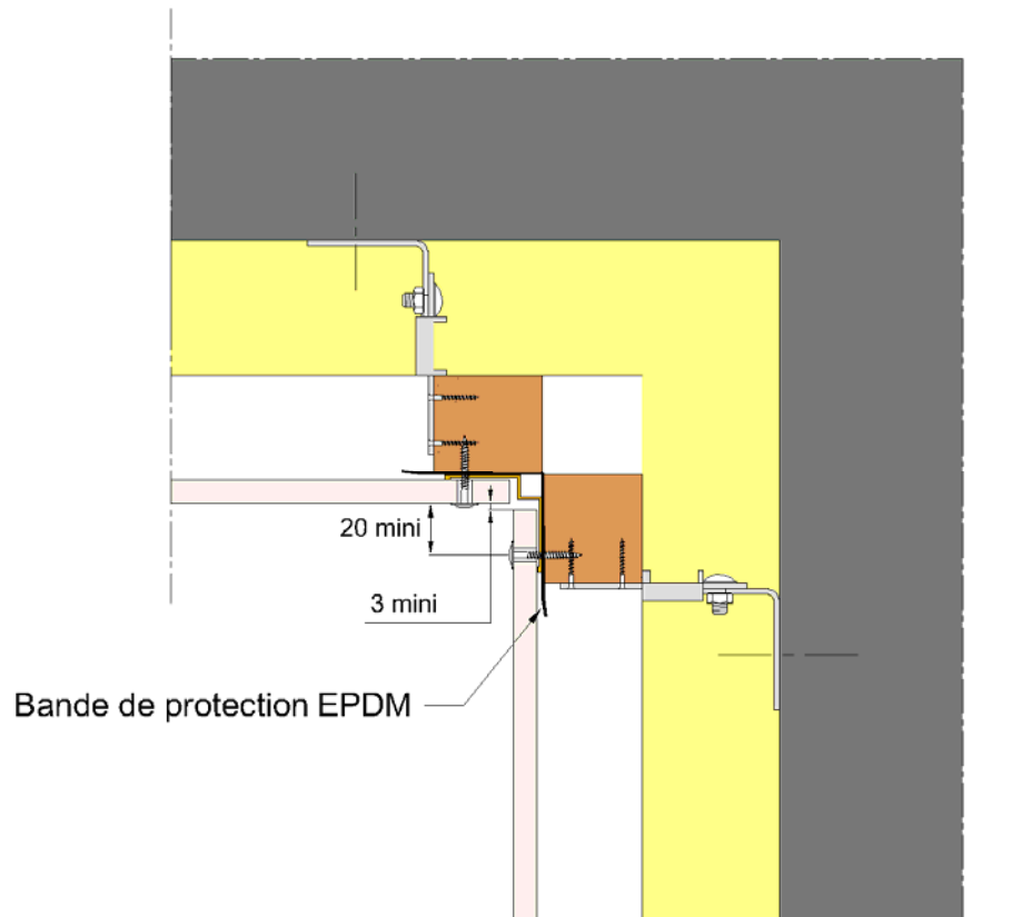
Figure 13bis – Angle rentrant (Cas des joints horizontaux fermés avec le profile PVC H)
