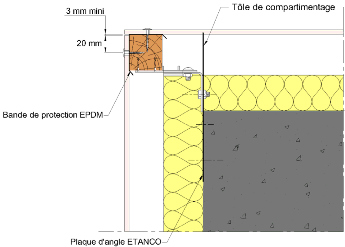
Figure 11bis - Angle sortant sans profilé (bardage)
