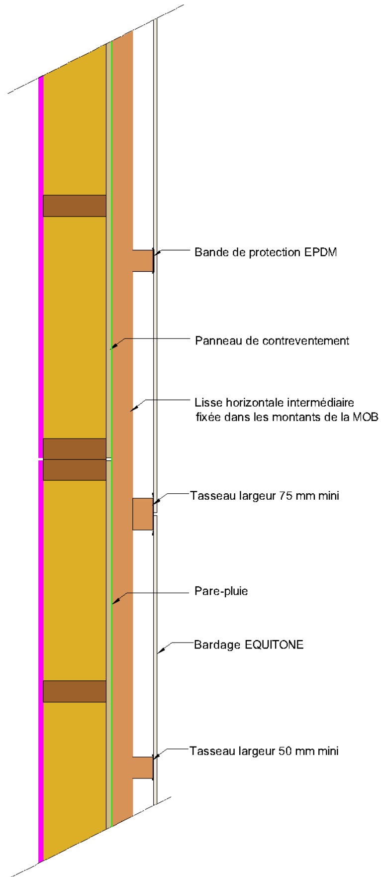
Figure 20 - Ossature croisée - Coupe horizontale - Pose sur COB
