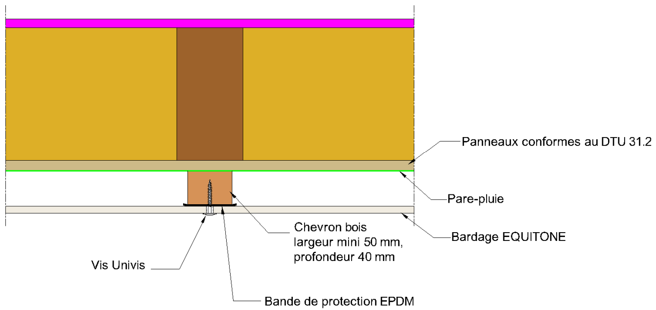
Figure 25 - Fixation intermédiaire de la plaque - Pose sur COB
