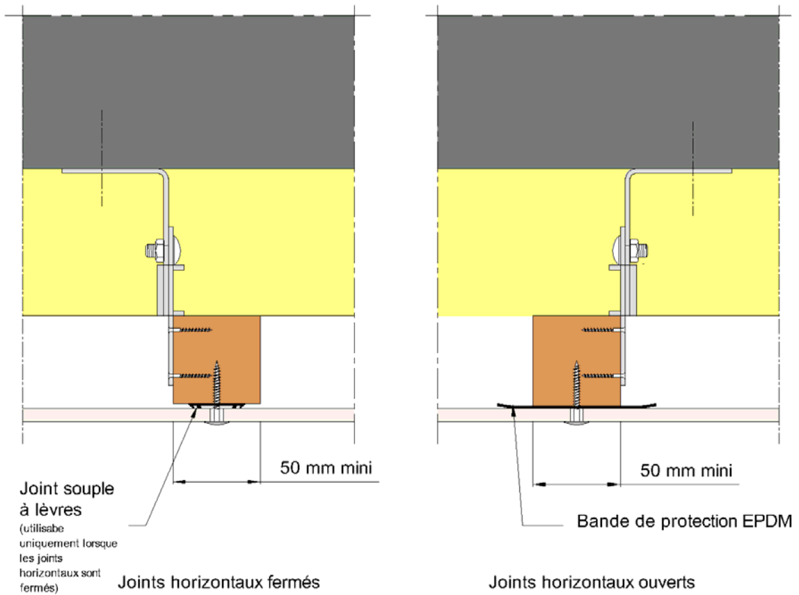
Figure 9 - Fixation sur chevron intermédiaire
