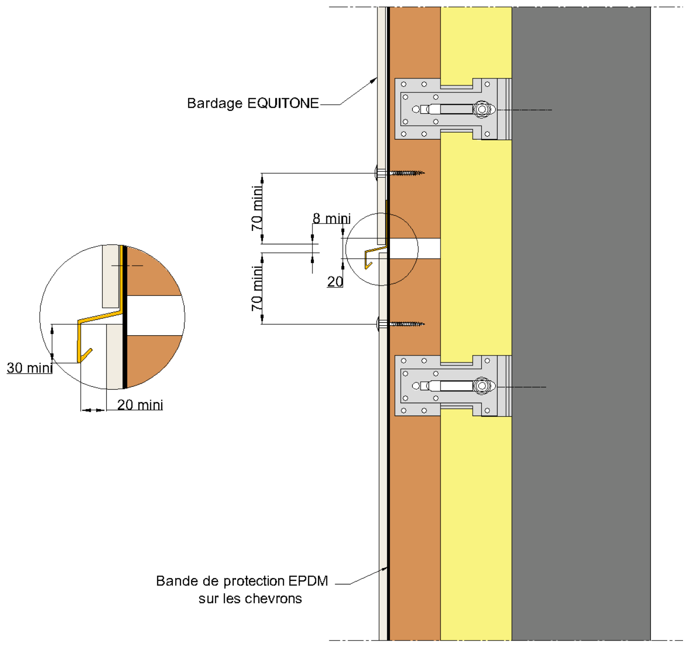
Figure 17bis- Fractionnement de l'ossature pour des chevrons d'une longueur comprise entre 5,4 m et 11 m
