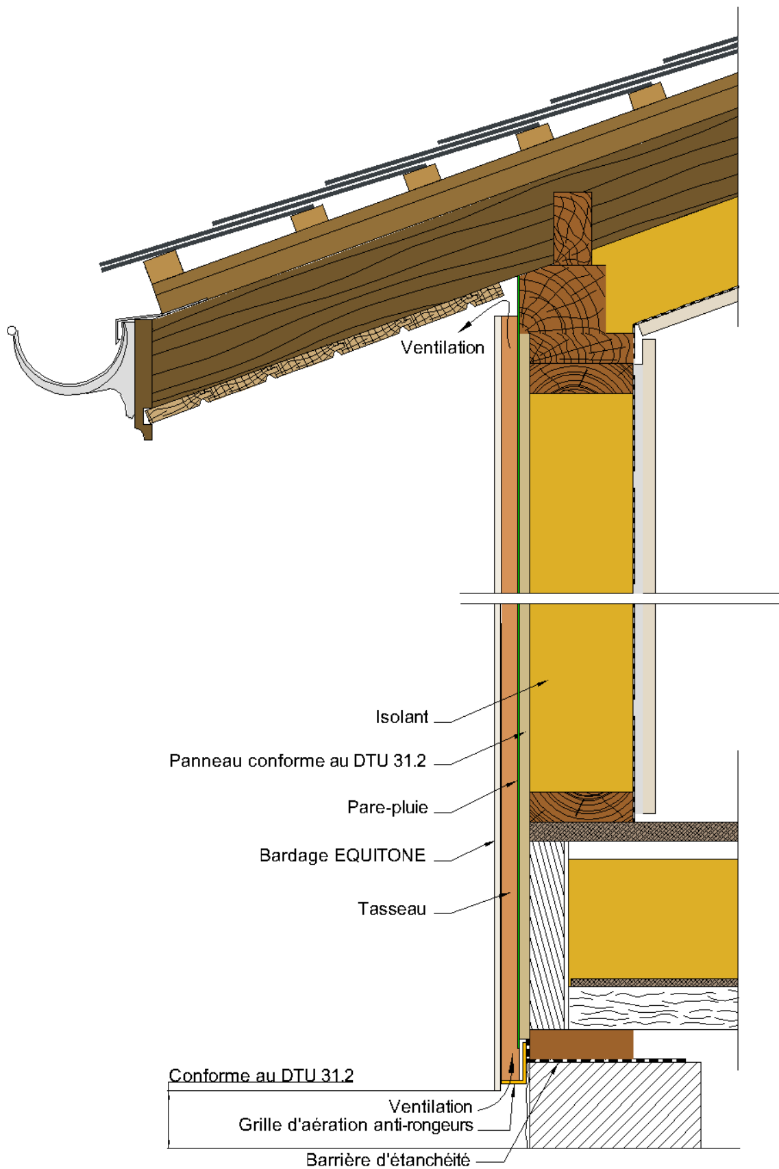
Figure 22 – Rive haute et rive basse - Pose sur COB
