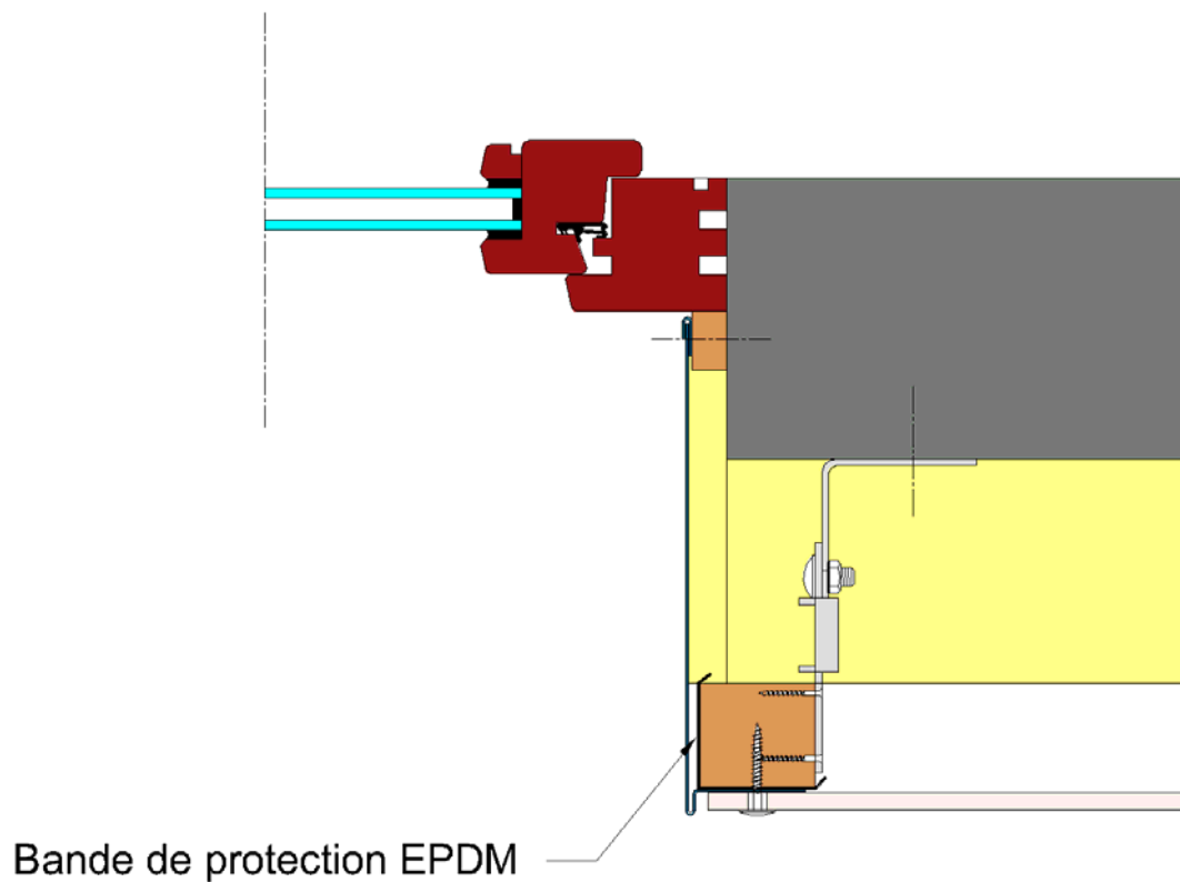
Figure 14 - Encadrement de fenêtre (coupe sur tableau)
