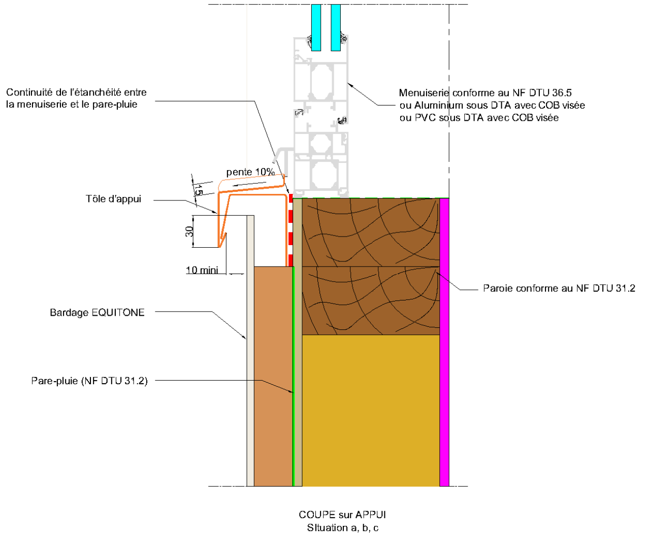
Figure 33 – Pose sur COB – Dispositions particulières du traitement des baies Menuiserie en tunnel au nu extérieur – Coupe sur appui de baie
