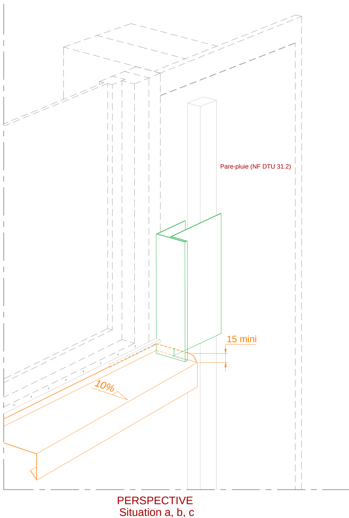
Figure 29 – Pose sur COB – Perspective Dispositions particulières du traitement des baies (Menuiserie en tunnel au nu extérieur)
