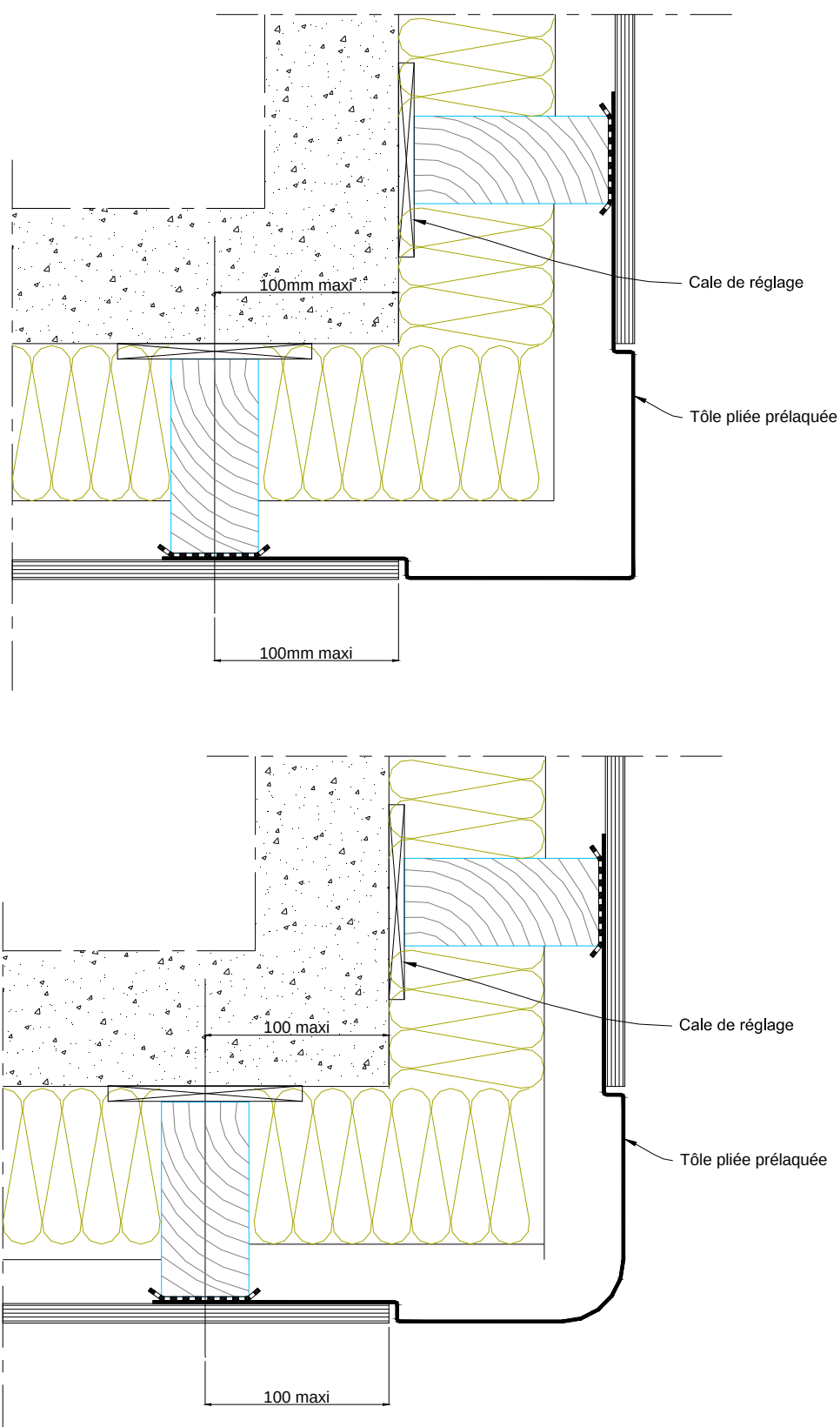
Figure 54 – Pose en zones sismiques directement sur support - Angle sortant
