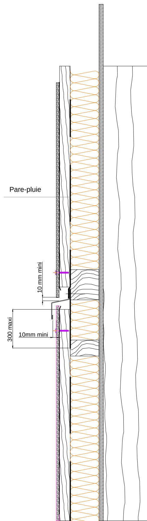
Figure 42 – Réseaux croisés sur COB - Recoupement du pare-pluie tous les 6 m avec le système multi-réseaux
