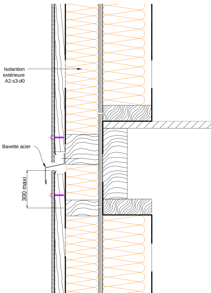
Figure 43 – Réseaux croisés sur COB - Fractionnement de la lame d'air pour respecter l'IT 249
