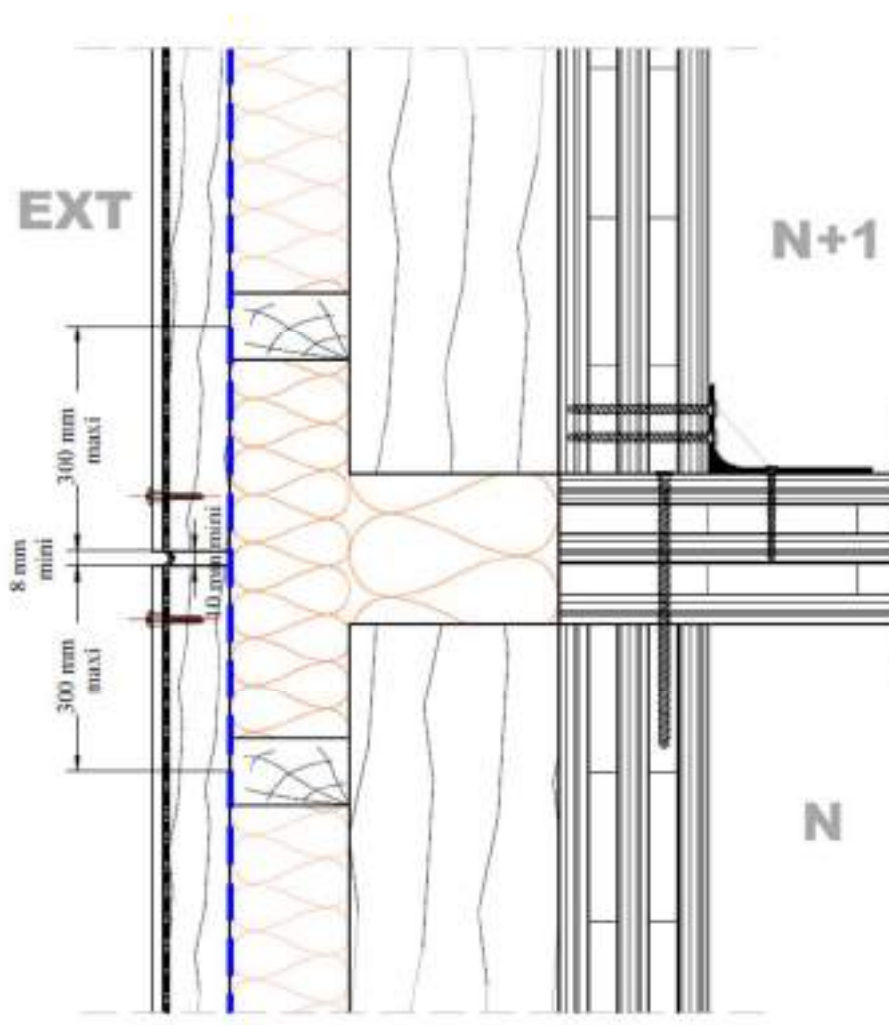
Figure 58 – Pose en zones sismiques directement sur support -Fractionnement de l'ossature au droit de chaque plancher CLT
