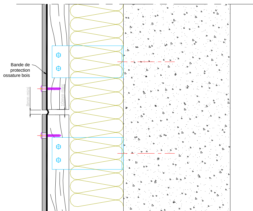
Figure 14 – Fractionnement de l'ossature Montants inférieurs à 5,40 m
