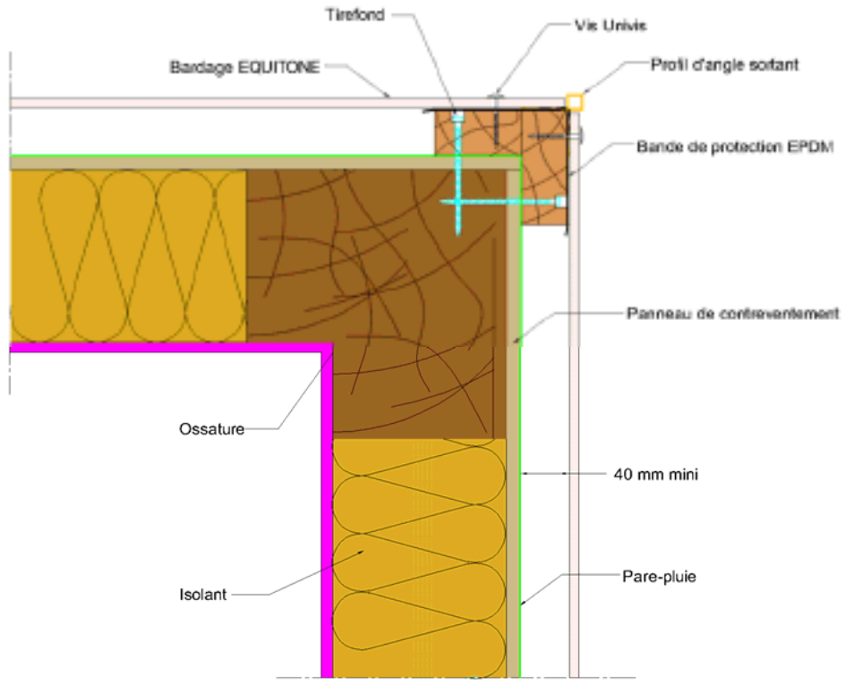
Figure 26 – Traitement de l'angle sortant – Pose sur COB
