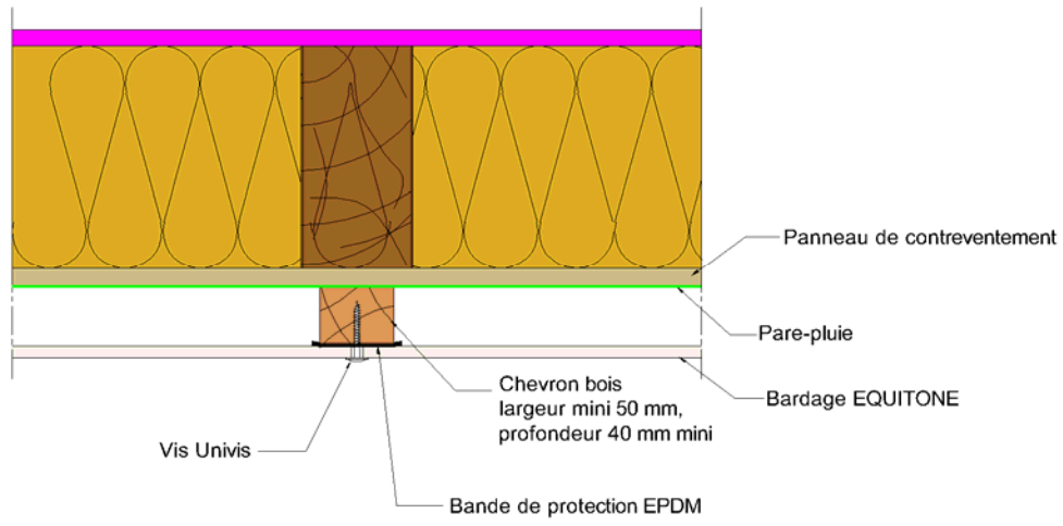
Figure 22 – Principe de fixation sur chevron intermédiaire – Pose sur COB
