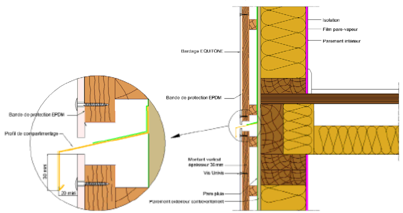
Figure 29 – Fractionnement au droit des planchers pour la COB – ossature croisée
