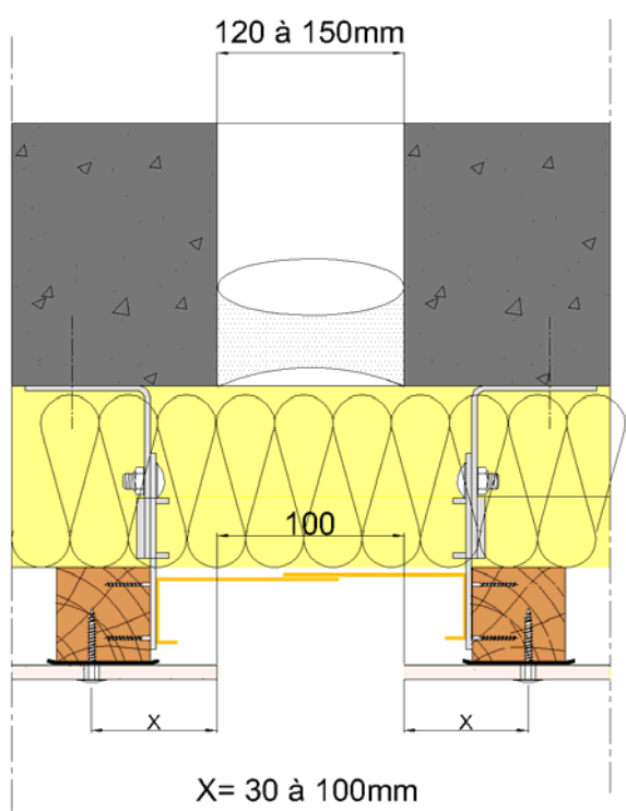
Figure 40 – Joint de dilatation de 120 à 150 mm
