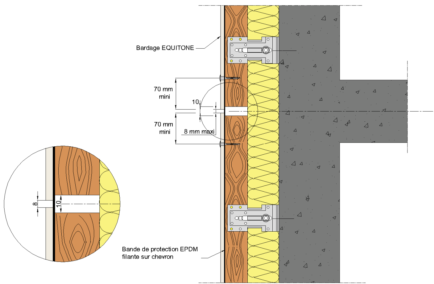
Figure 38 - Fractionnement de l'ossature bois au niveau du plancher
