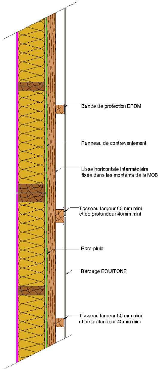
Figure 19 - Ossature croisée - Pose sur COB (Coupe horizontale)
