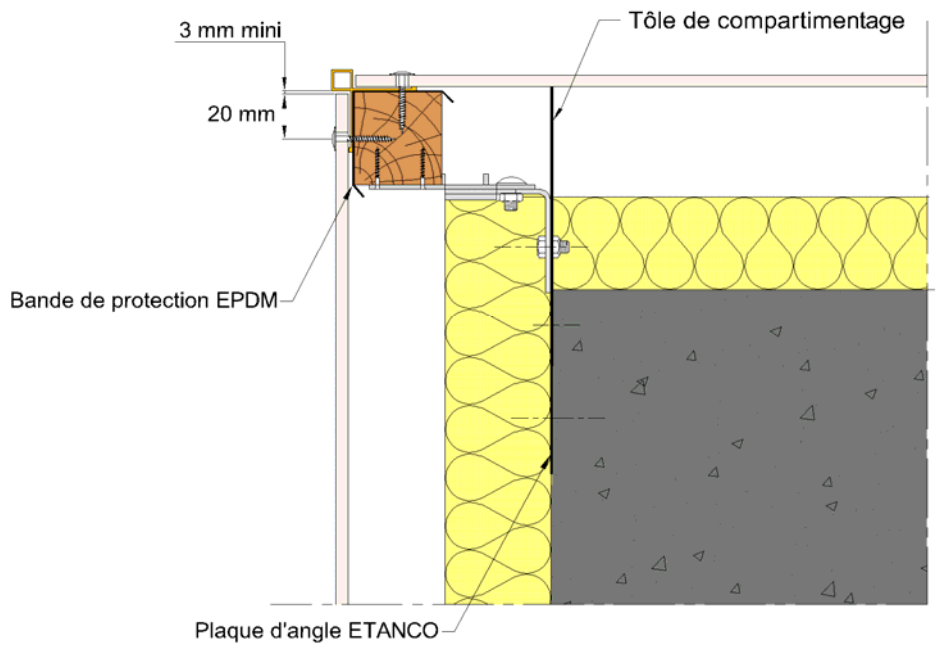
Figure 10 - Angle sortant avec profilé
