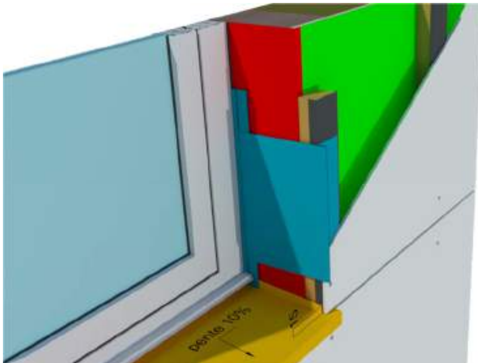
Figure 33 – Pose sur COB – Perspective Dispositions particulières du traitement des baies (Menuiserie en tunnel intérieur)
