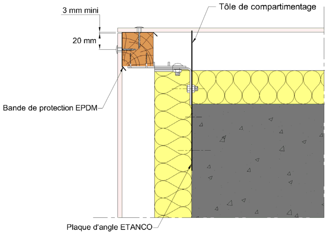
Figure 11bis - Angle sortant sans profilé (sans bardage)
