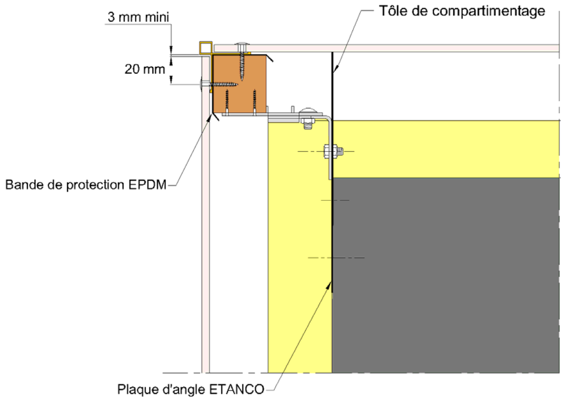
Figure 11 - Angle sortant avec profilé (bardage)
