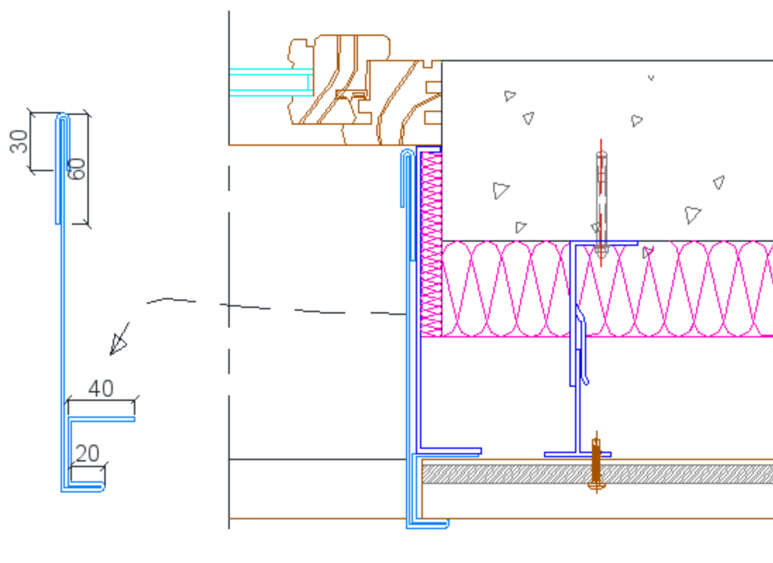
Figure 32 – Tableau de baie en pose horizontale
