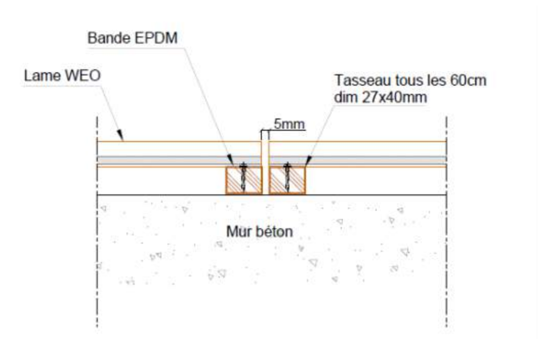
Figure 7bis – Jonction de lame - Coupe horizontale
