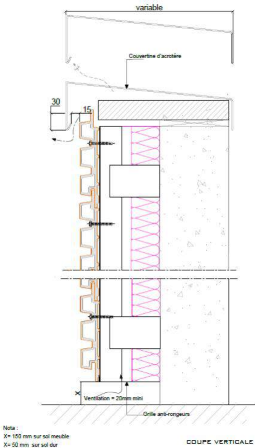
Figure 28 – Départ et arrêt haut bardage sur ossature métallique en pose horizontale - Coupe verticale
