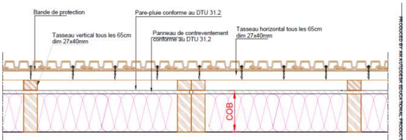
Figure 43 – Coupe horizontale – Pose verticale sur COB
