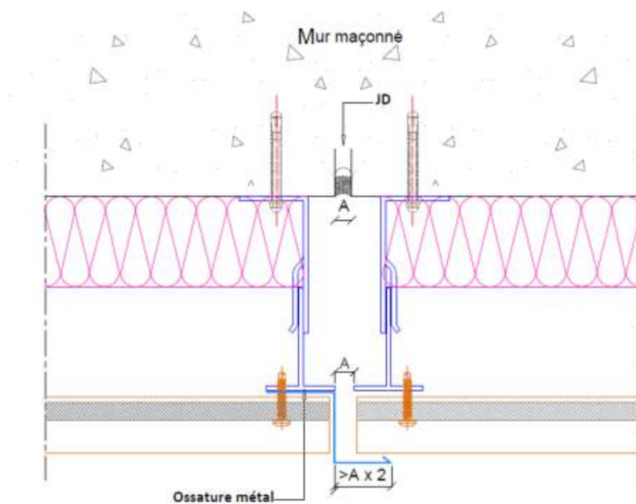
Figure B2– Détail joint de dilatation de 12 à 15 cm
