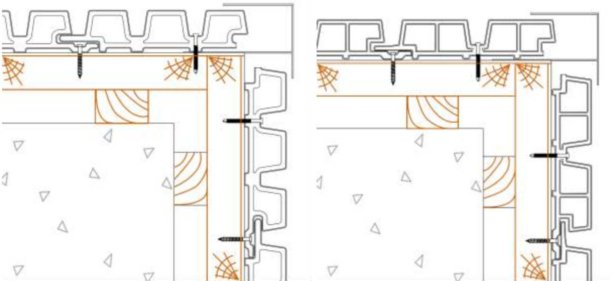
Figure 47 – Angle sortant en vissage invisible en pose verticale
