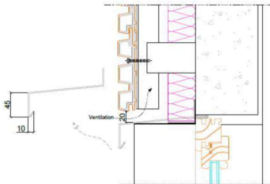
Figure 30 – Linteau de baie en pose horizontale
