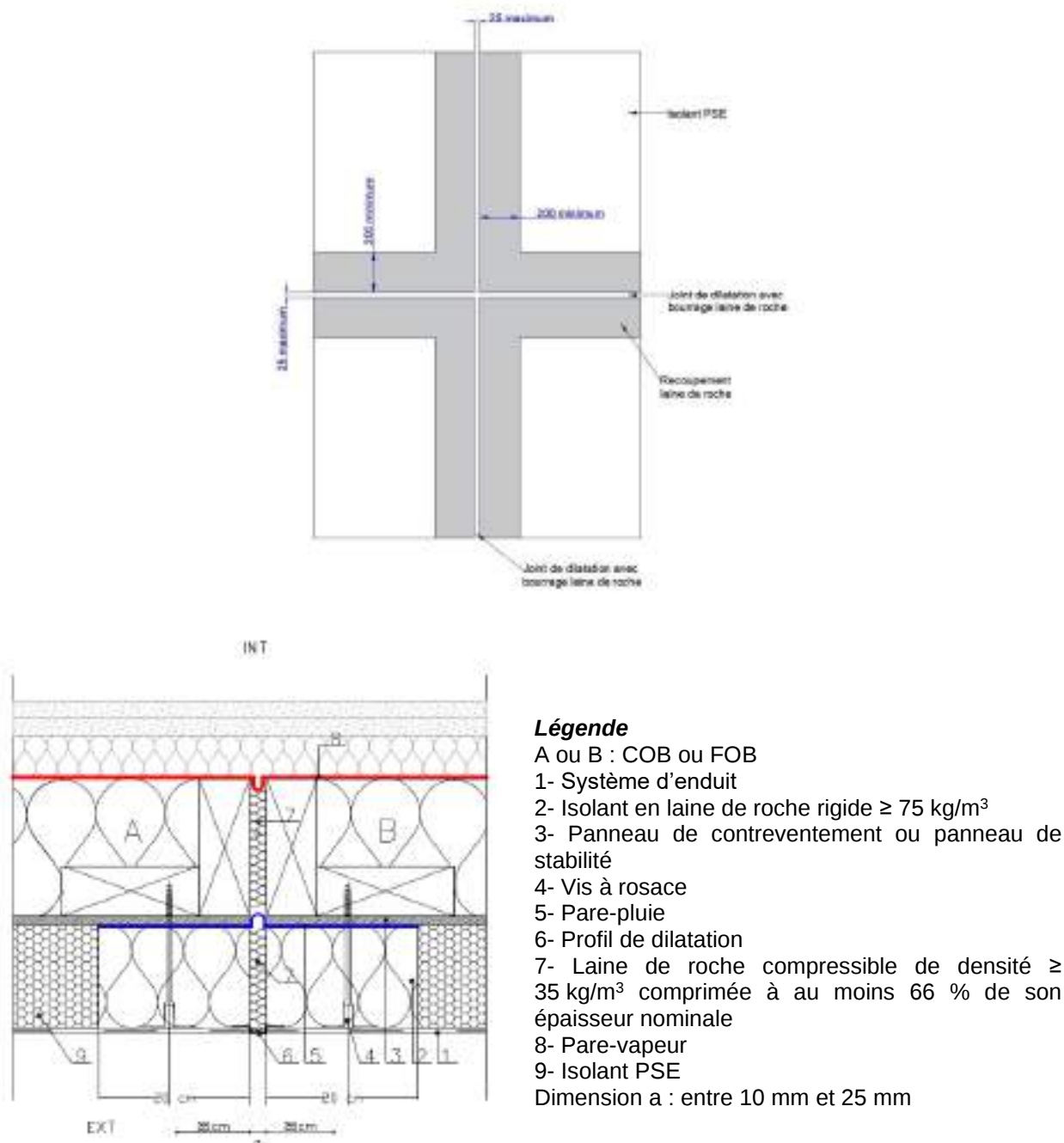
Figure 9 : Dispositions générales pour les joints de dilatation
