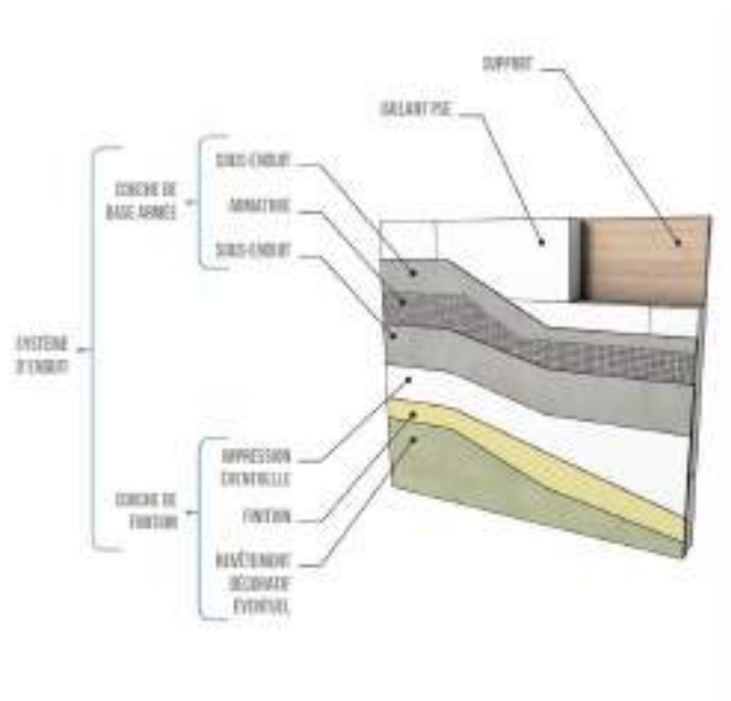
Figure 1 : Système isolation par l'extérieur par enduit sur PSE (fixation de l'isolant non représentée)
