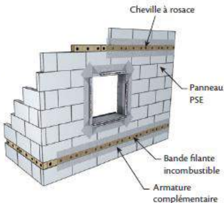
Figure 2 : protection incendie par bandes filantes incombustibles (crédit : [5])
