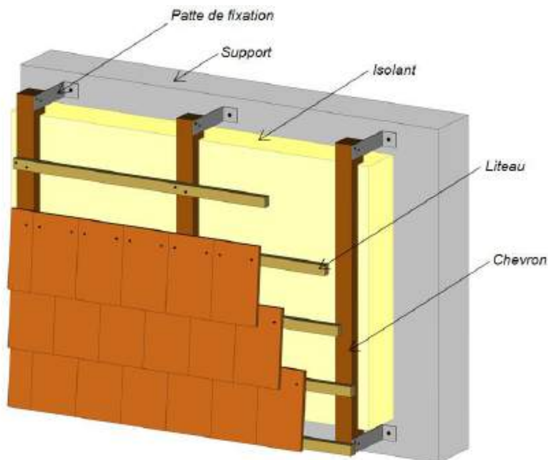
Figure n° 1 : Mise en œuvre sur façade de type A et B
