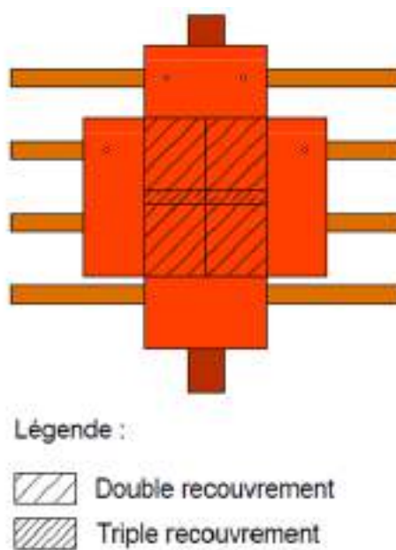
Figure n° 3 : Principe de mise en œuvre de tuiles plates en pose jointive
