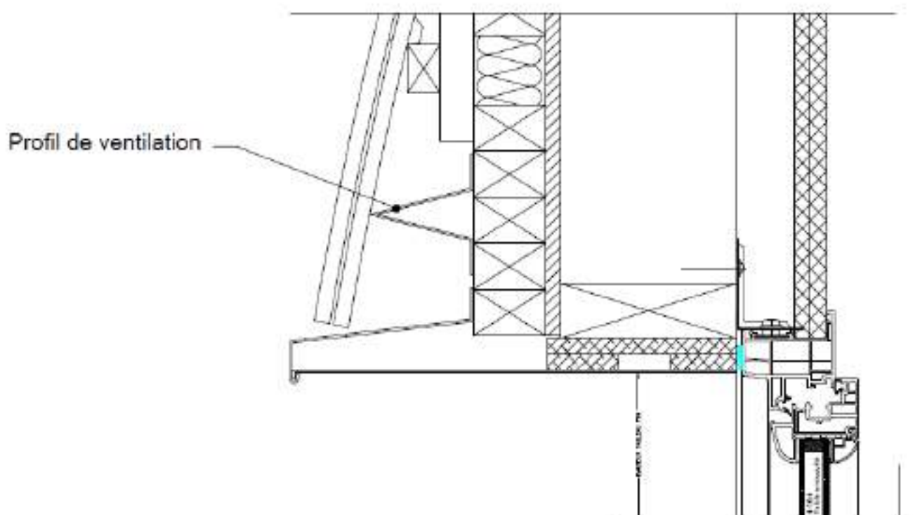
Figure n° 7 : Mise en œuvre du profilé de ventilation en linteau de baie
